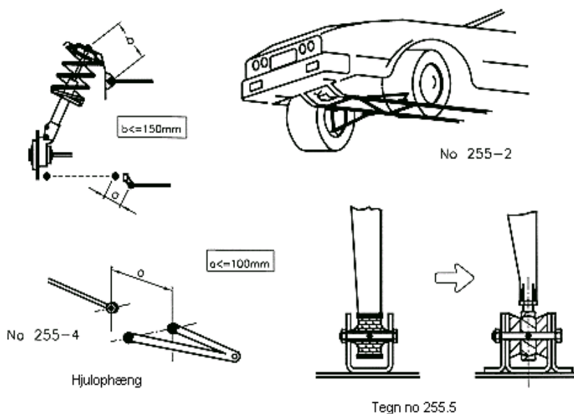
Tilladte ændringer i hjulophæng og undervogn
